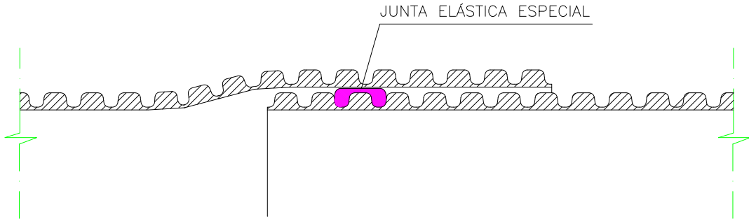
DETALLE JUNTA ELÁSTICA ESCALA: S/E
