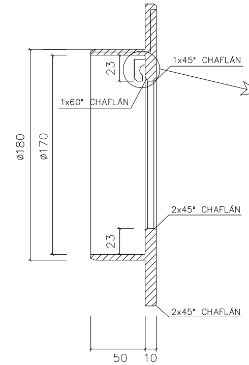
SECCIÓN A-A'
