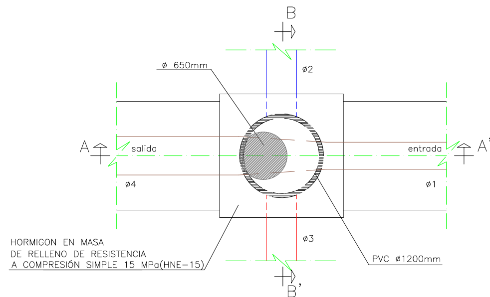
PLANTA
