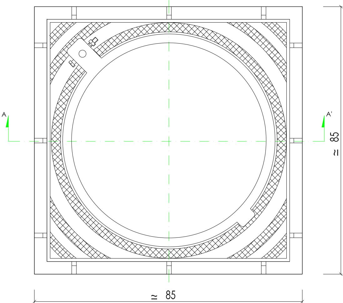
PLANTA - EMPLEAR EN ACERA
