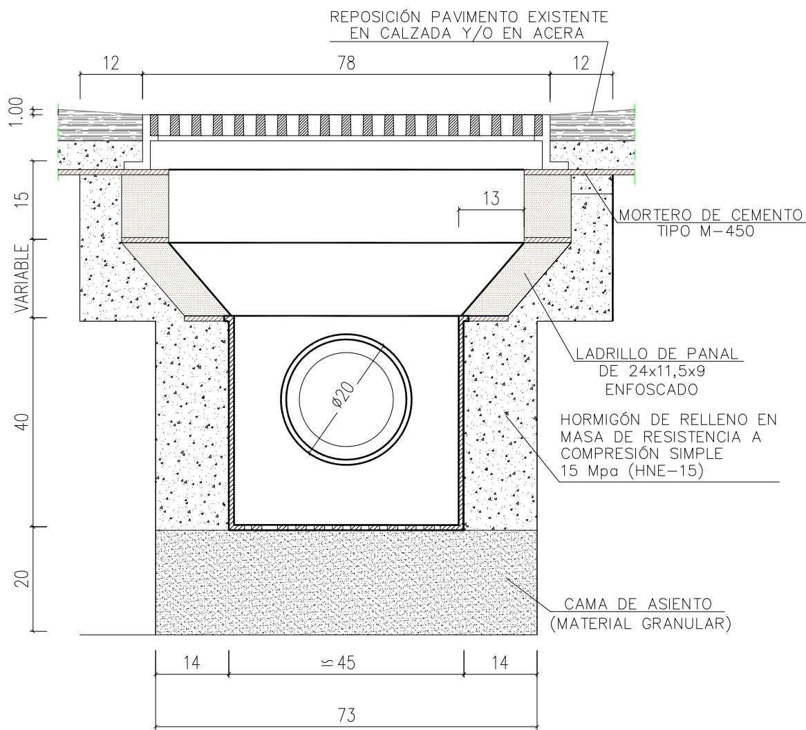
SECCIÓN A-A'
