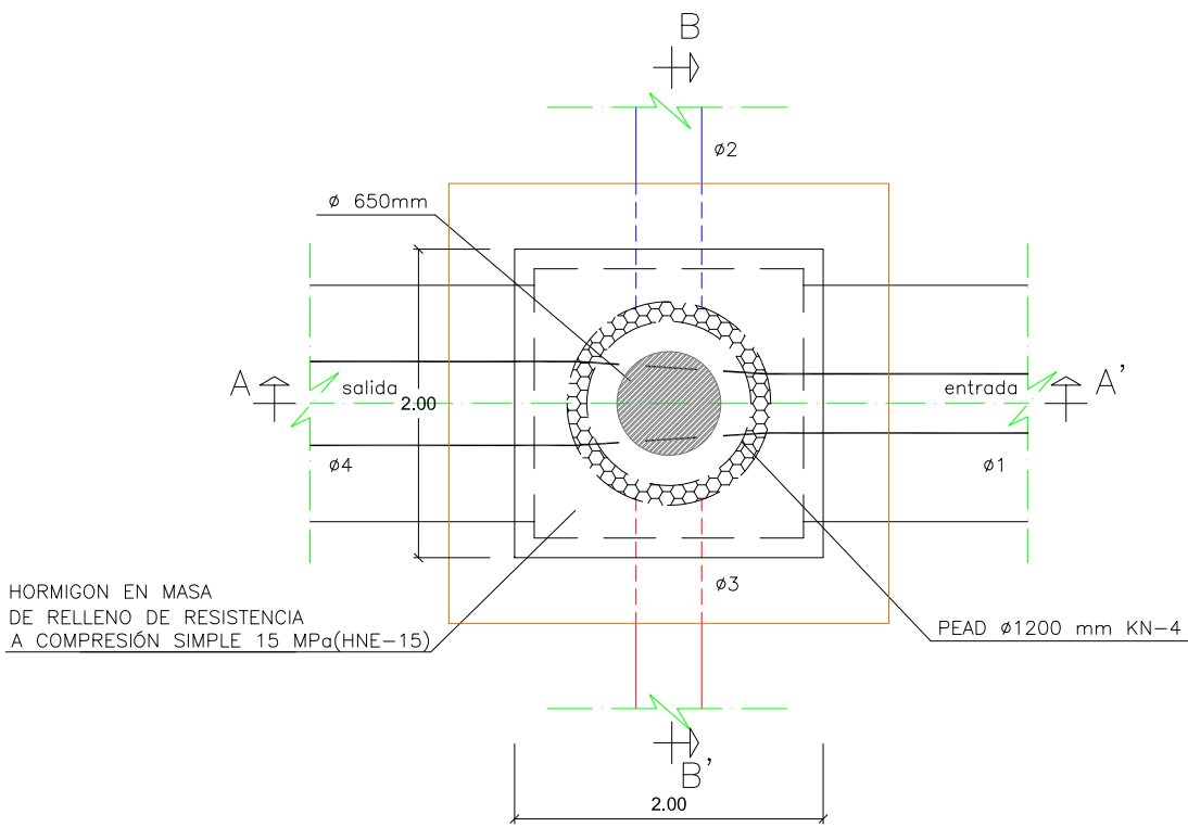
PLANTA
