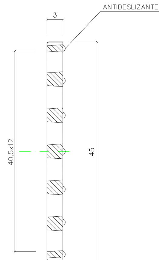
SECCIÓN B - B'
