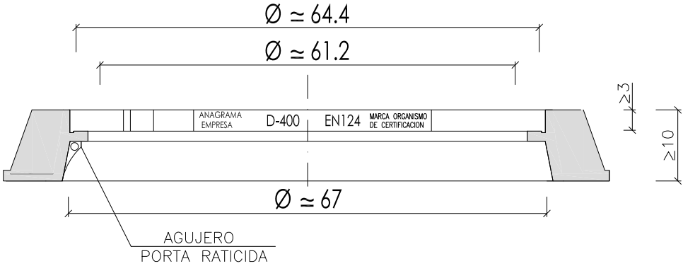
SECCIÓN A-A'
