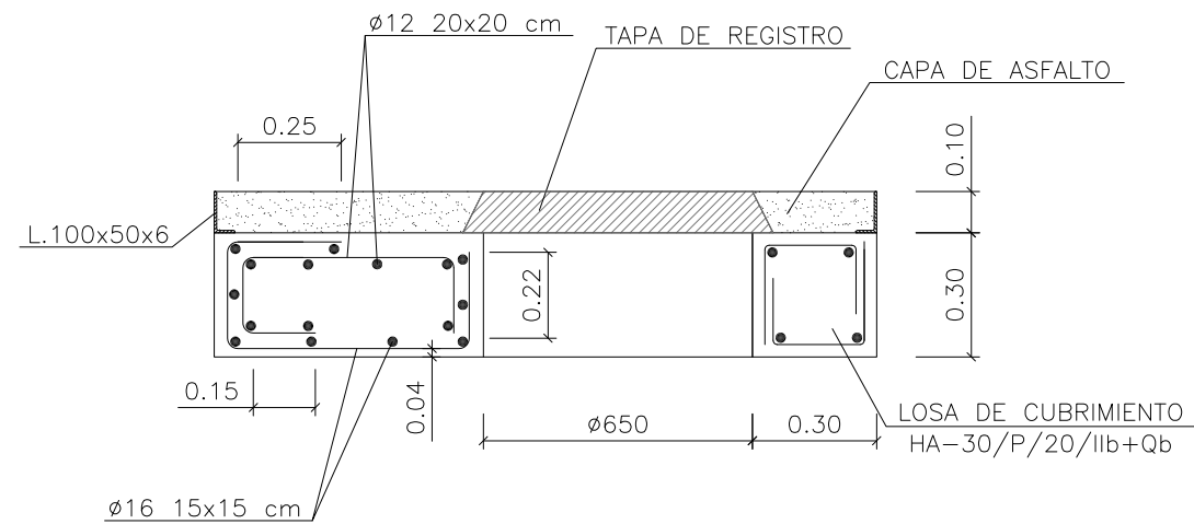
SECCIÓN A-A'
