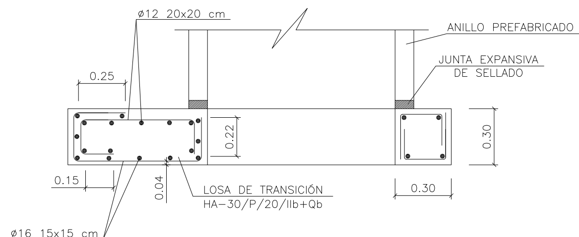
SECCIÓN B-B'
