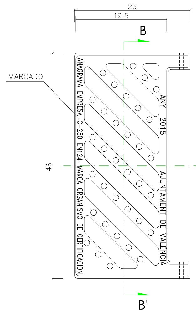
PLANTA
