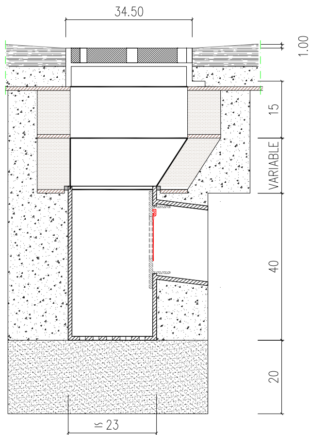
SECCIÓN B-B'
