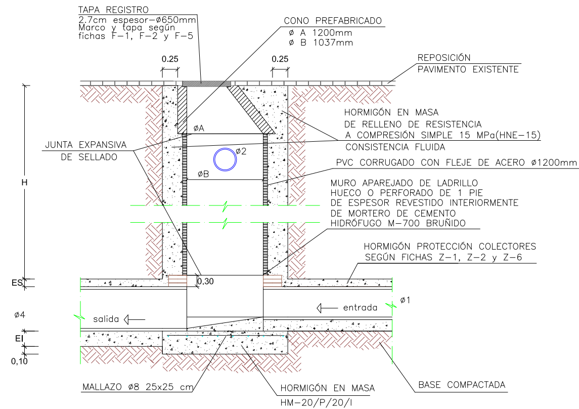
SECCIÓN A-A'
