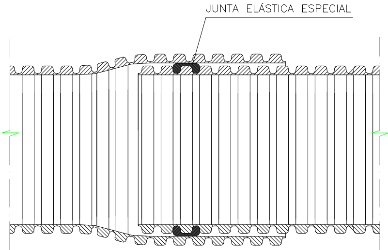
DETALLE JUNTA ELÁSTICA ESCALA: S/E
