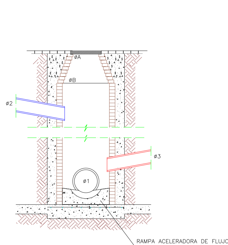
SECCIÓN B-B'
