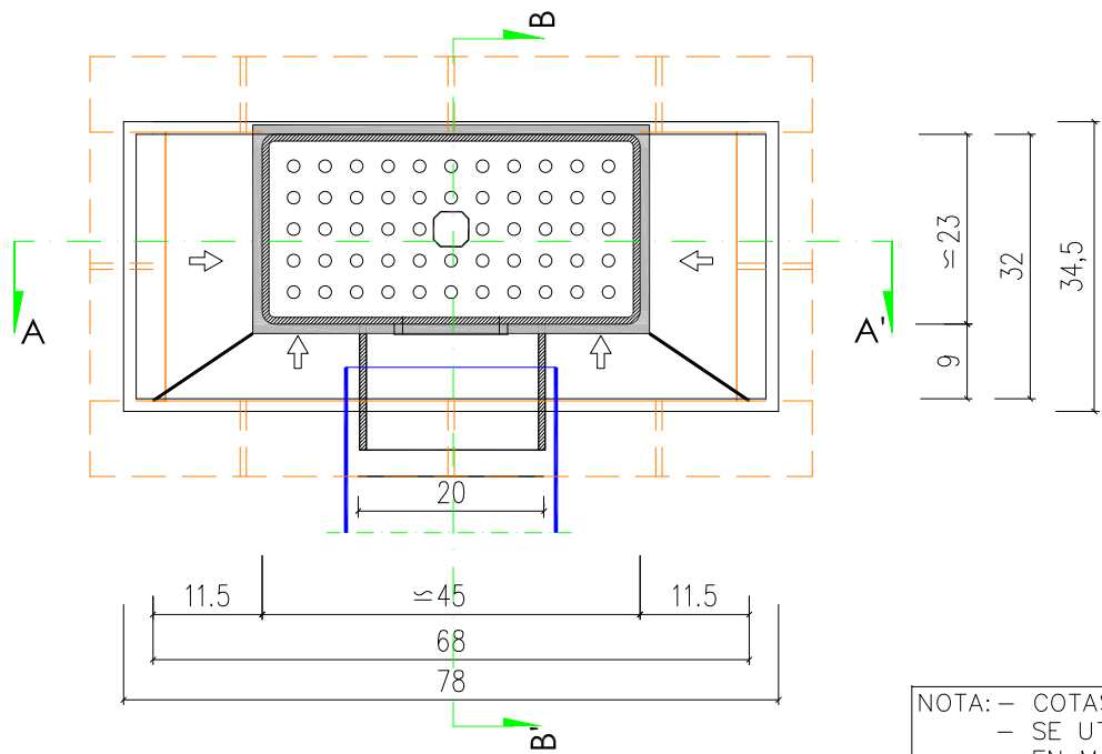
PLANTA
