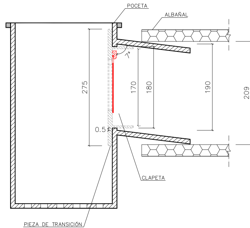
POSICIÓN EN POCETA
