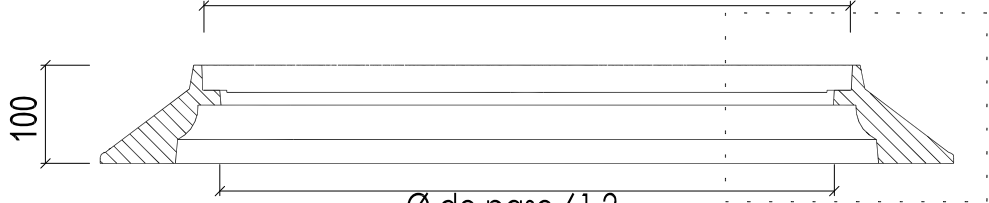
SECCIÓN B-B Ø de paso 61.2
