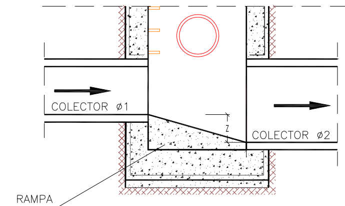
DETALLE 1 SECCIÓN A-A' ARQUETÓN VISITABLE
