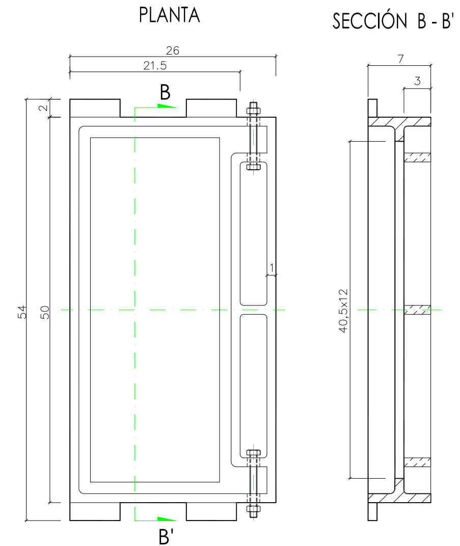
TORNILLERÍA (S/E)
