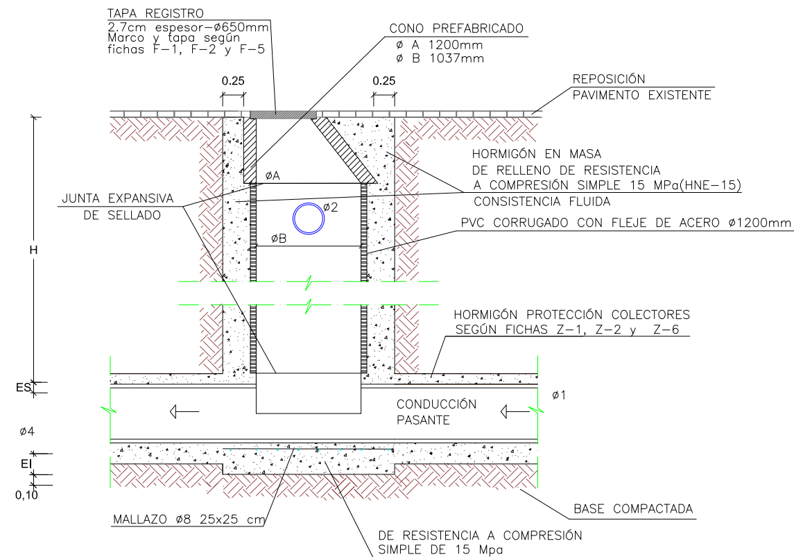
SECCIÓN A-A'
