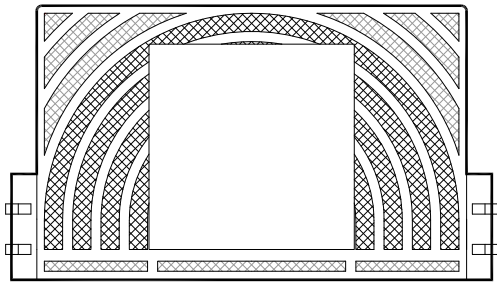
IMBORNAL "VALENCIA". MARCO
