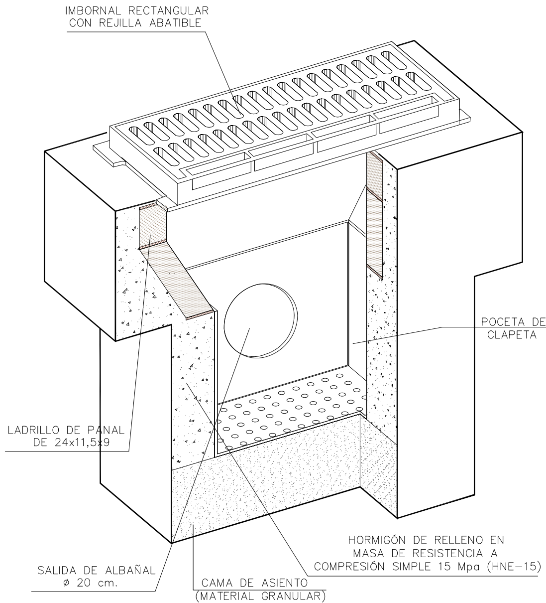
PERSPECTIVA
