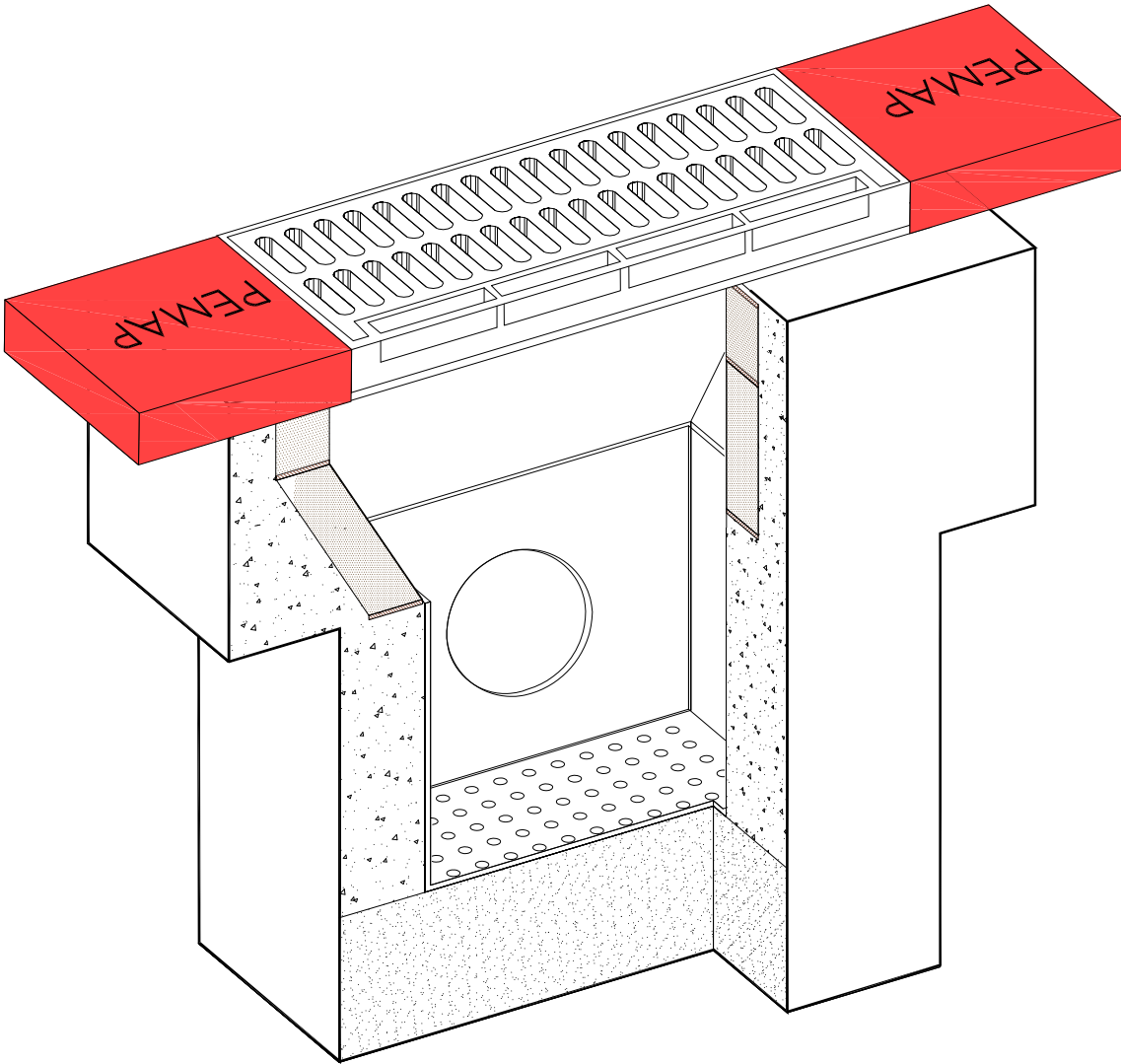
SUMIDERO RECTANGULAR 78 cm.
