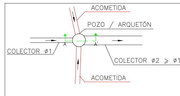
ESQUEMA PLANTA
