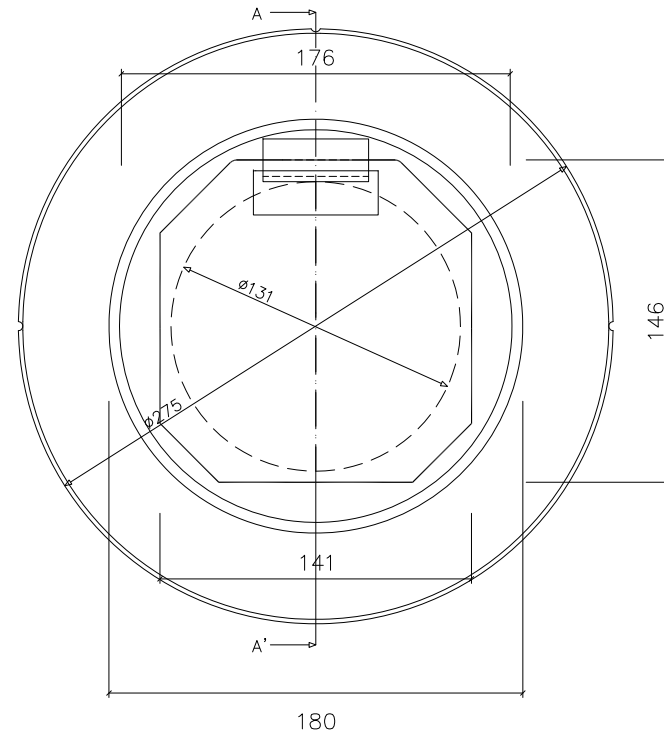
PIEZA DE TRANSICIÓN
