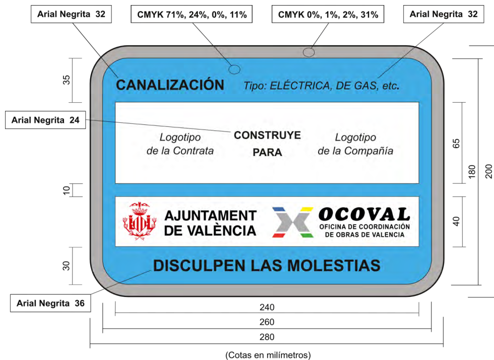
Figura 2. Cartel de obra para colocación en vallas
