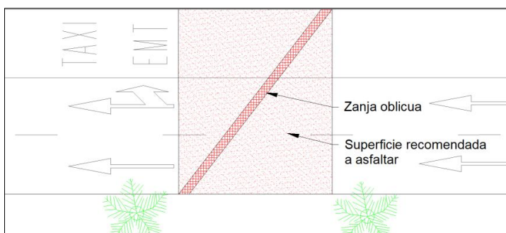
Figura 3. Afección varios carriles. Superficie recomendada.
