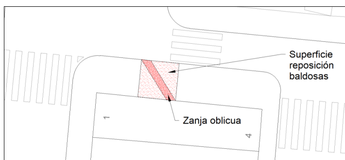
Figura 6. Superficie reposición baldosas en zanja oblicua.
