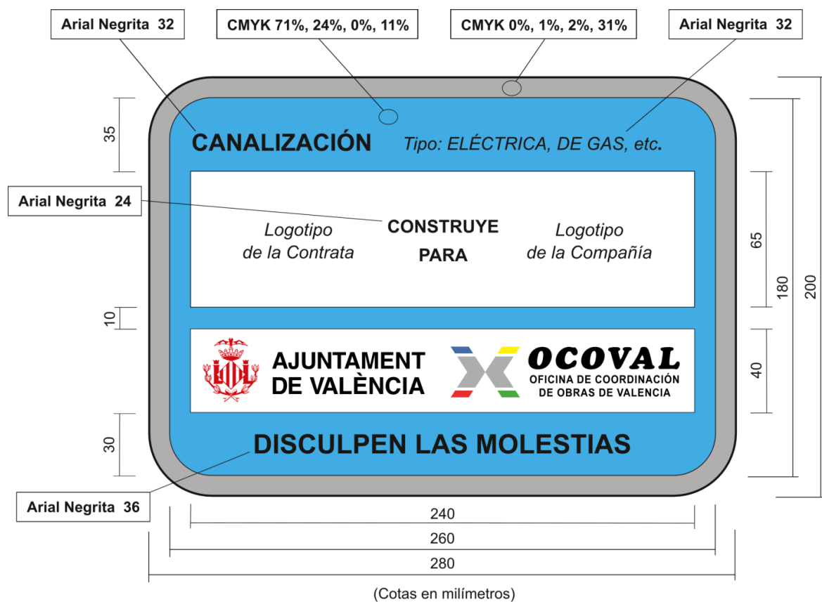
Figura 2. Cartel de obra para colocación en vallas
